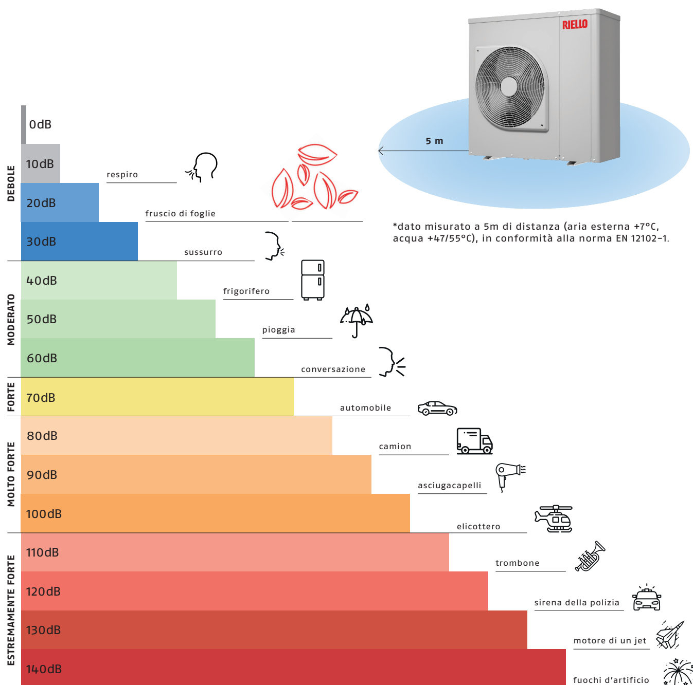
Scala delle emissioni sonore percepite in dB con esempi di livelli compresi tra 0 e 140 dB.
