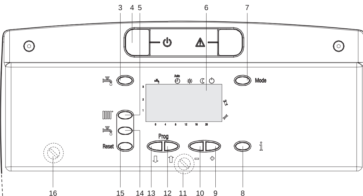
QUADRO DI COMANDO IN POSIZIONE APERTA
