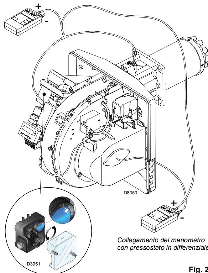
Collegamento del manometro con pressostato in assoluto
