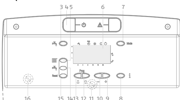
QUADRO DI COMANDO IN POSIZIONE APERTA
