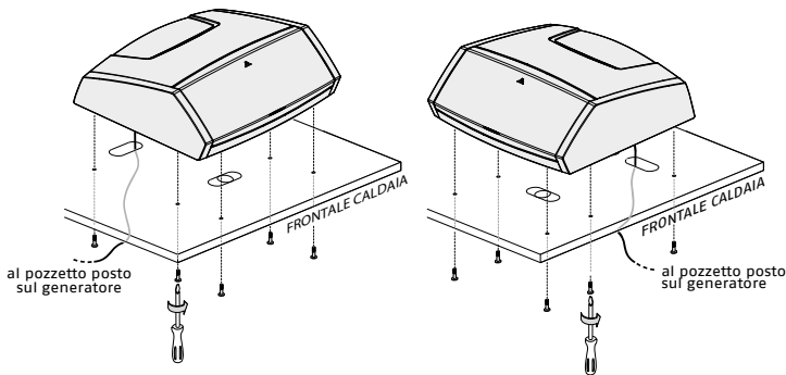
INSTALLAZIONE ORIZZONTALE
