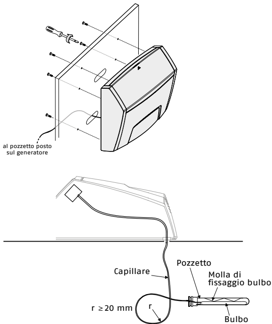
INSTALLAZIONE VERTICALE
