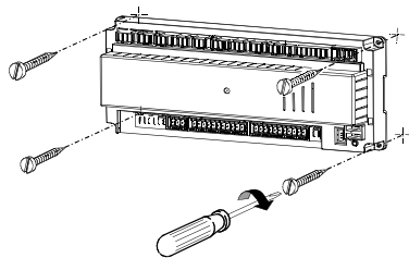
FISSAGGIO VITE
