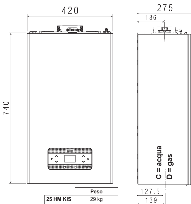
Dimensioni d'ingombro
