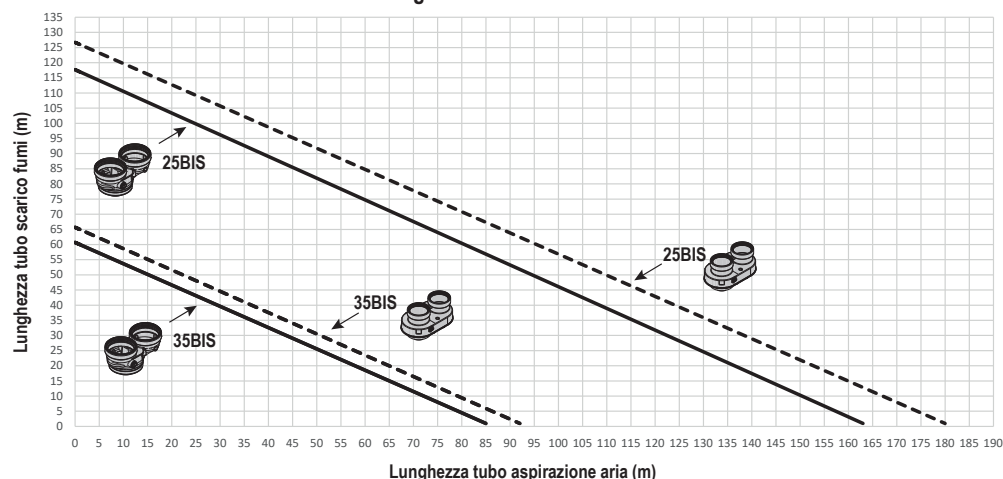
Lunghezza massimi tubi Ø 80 mm
