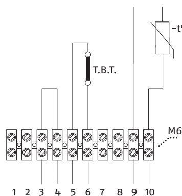
T.B.T. Termostato bassa temperatura S.E. Sonda esterna
