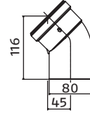
Curva 45°
