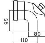
Curva 90° ispezionabile
