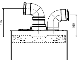
CONDOTTI SDOPPIATI Ø80-80
