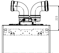
CONDOTTI SDOPPIATI Ø80-80 CON ADATTATORE COMPATTO
