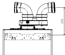
CONDOTTI SDOPPIATI Ø80-80 CON ADATTATORE
