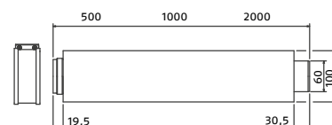
Prolunga
