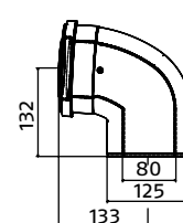
Curva 90°
