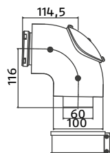
Curva 90° ispezionabile
