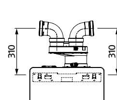
Ø80-80 con adattatore
