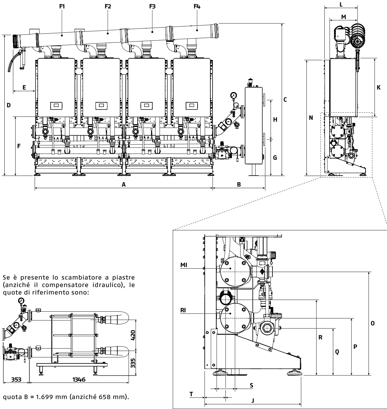
Disposizione in linea (FRONT) 4 moduli - [35-45kW]
