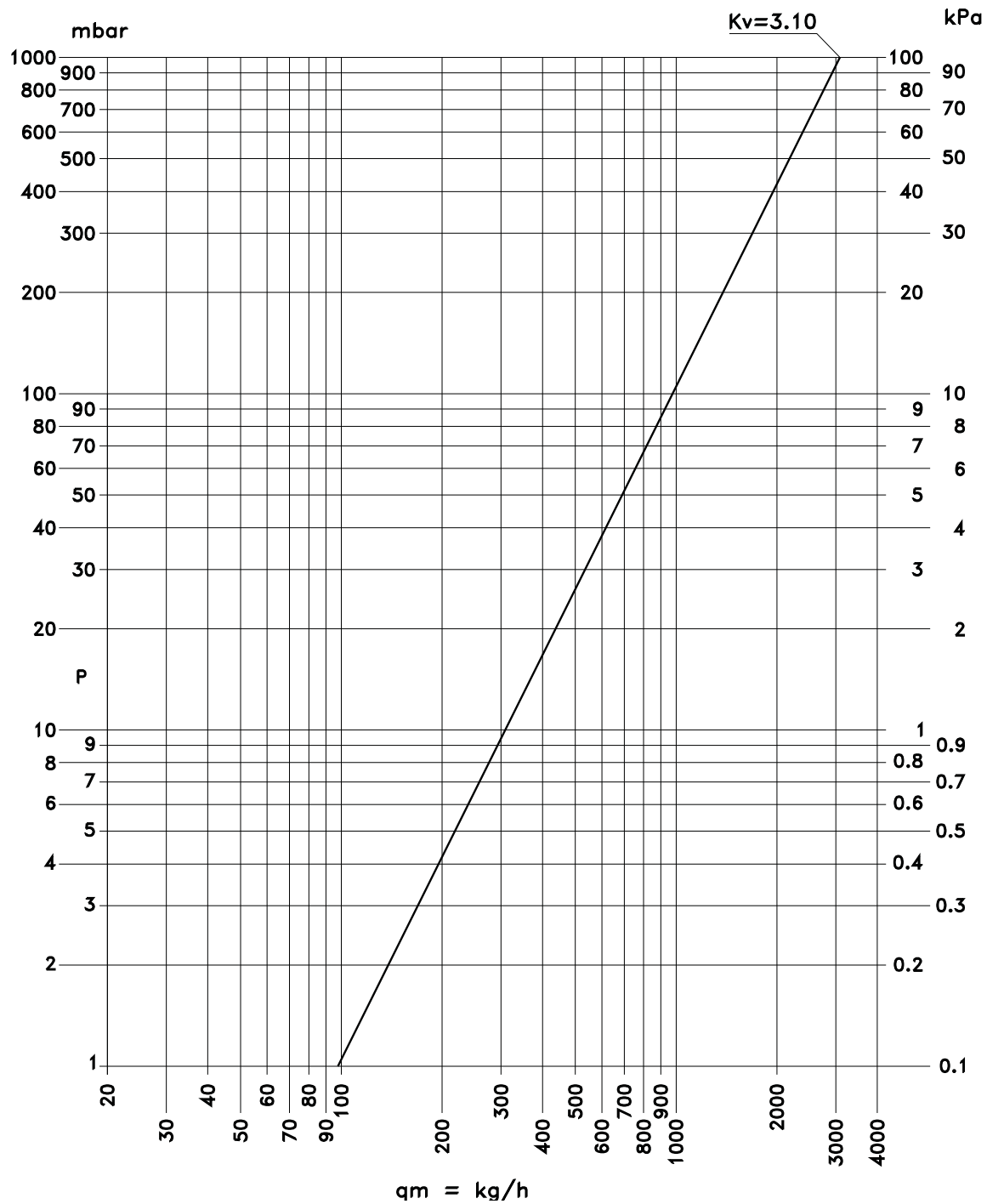
Diagramma perdite di carico valvola deviatrice in posizione tutta chiusa
