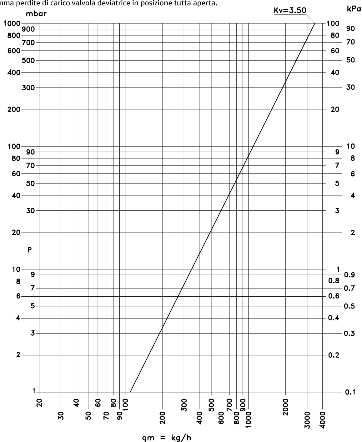
Diagramma perdite di carico valvola deviatrice in posizione tutta aperta.
