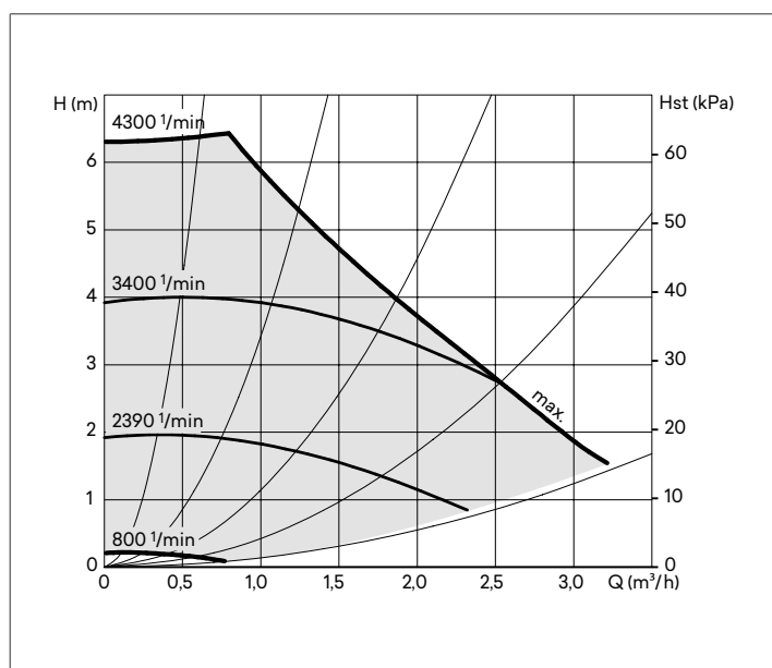
Grafico portata/prevalenza pompa circuito solare PP7
