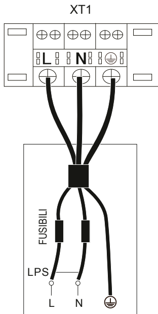
ALIMENTAZIONE UNITÀ INTERNA Resistenza elettrica monofase da 3kW standard
