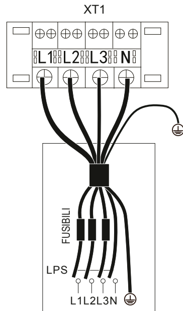
ALIMENTAZIONE UNITÀ INTERNA Resistenza elettrica trifase da 9kW standard
