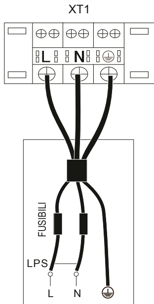
ALIMENTAZIONE UNITÀ INTERNA Resistenza elettrica monofase da 4kW standard
