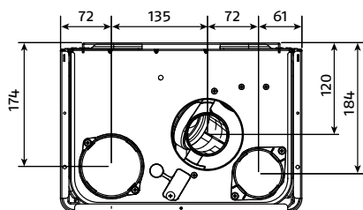
Vista dall'alto
