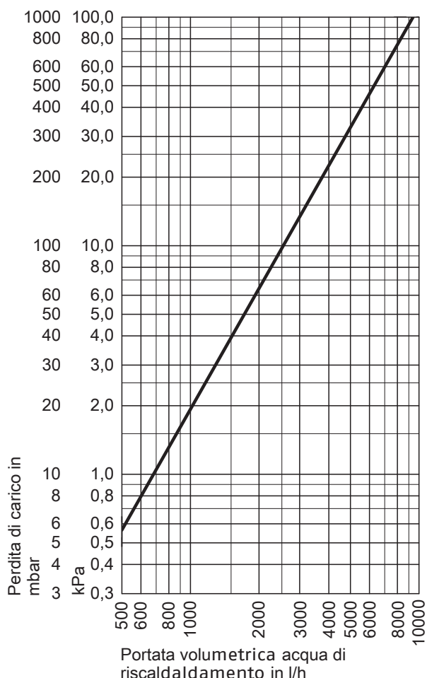
Perdita di carico lato riscaldamento serpentino per fonte ausiliaria di calore (solo tipo NEXPRO 250 S ACS)
