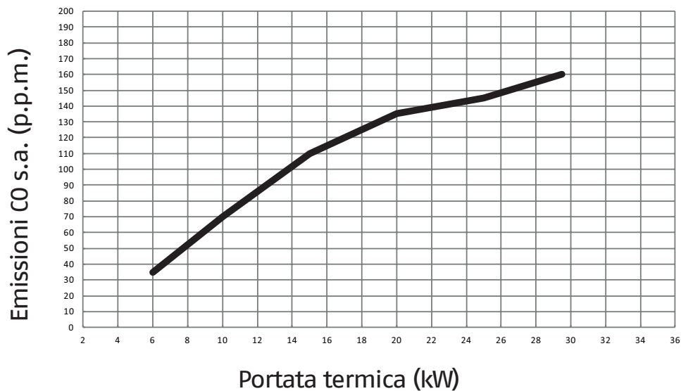
Curva portata termica - emissioni
