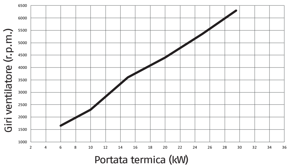
Curva portata termica - giri ventilatore
