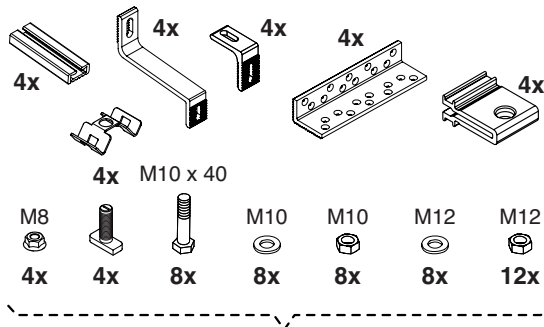
Sistem za fiksiranje na krov (D) Sistem za pritrditev na streho (D)
