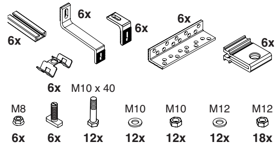
System voor bevestiging aan het dak (E) Sistema para la fijación en tejados (E)
