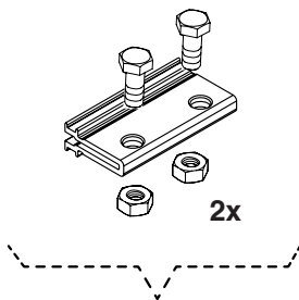
Pièces de liaisons (E) (si nécessaires) Verbindungsblaschen (F) (sofern erforderlich)
