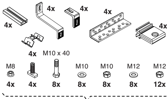
Sistema per il fissaggio al tetto (D) Roof fixing system (D)
