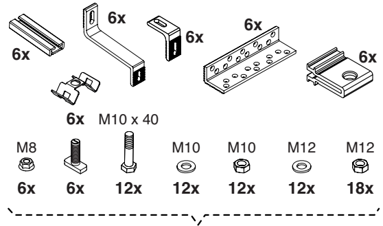
Système de fixation au toit (E) Dach-Befestigungssystem (E)
