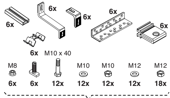
Sistema per il fissaggio al tetto (E) Roof fixing system (E)
