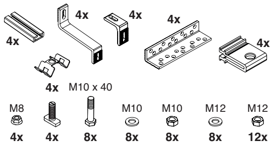
System voor bevestiging aan het dak (D) Sistema para la fijación en tejados (D)
